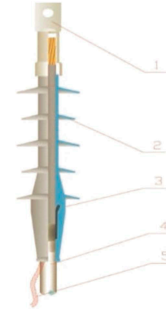
Концевая муфта наружной установки холодной усадки(15/24/35кВ)
