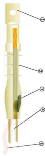
Концевая муфта внутренней установки холодной усадки(15/24/35кВ)
