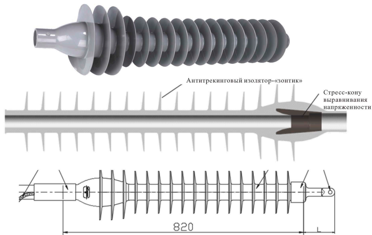
66 кВ Концевая муфта наружной установки в сборе
